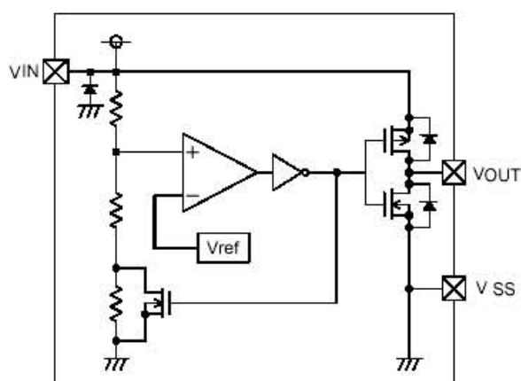
(1) CMOS Output
