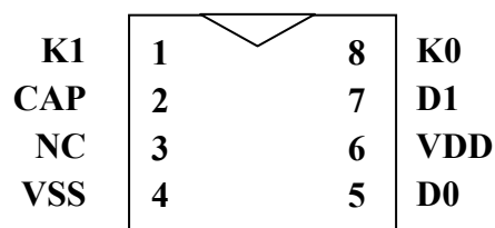
SG2908 SOP8
