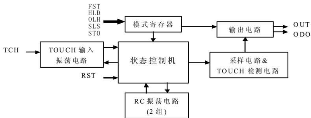
图 1 功能模块图
