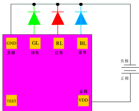
应用原理图
