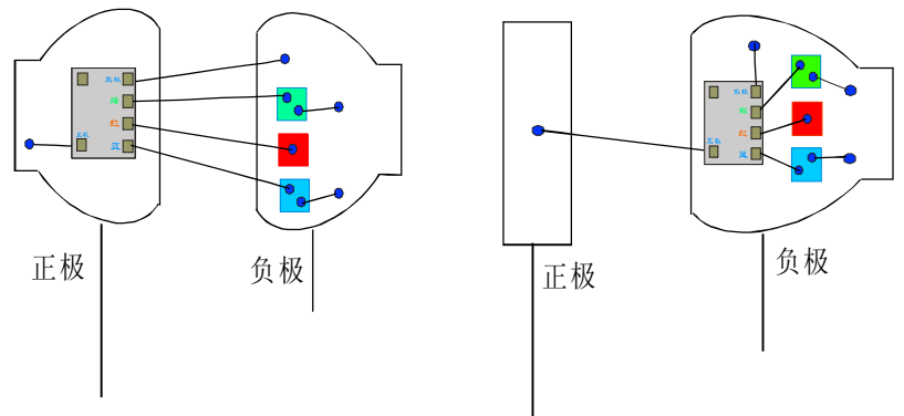
支架焊线图
