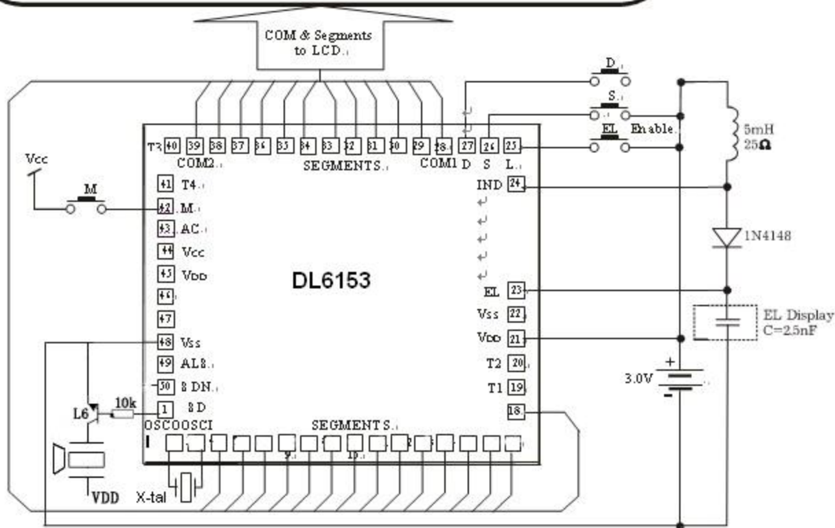
防止接蜂鸣片时白板的接法,加L6和10K电阻
