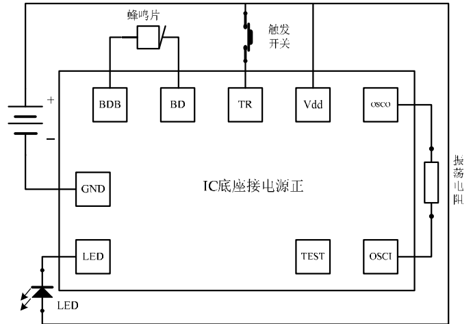
外接振荡电阻应用图
