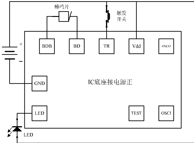
内置振荡电阻应用图
